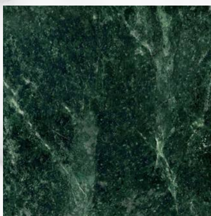
Мрамор Змеевик
